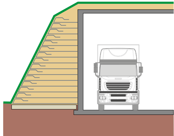
Mascheramento strutture in c.a.
