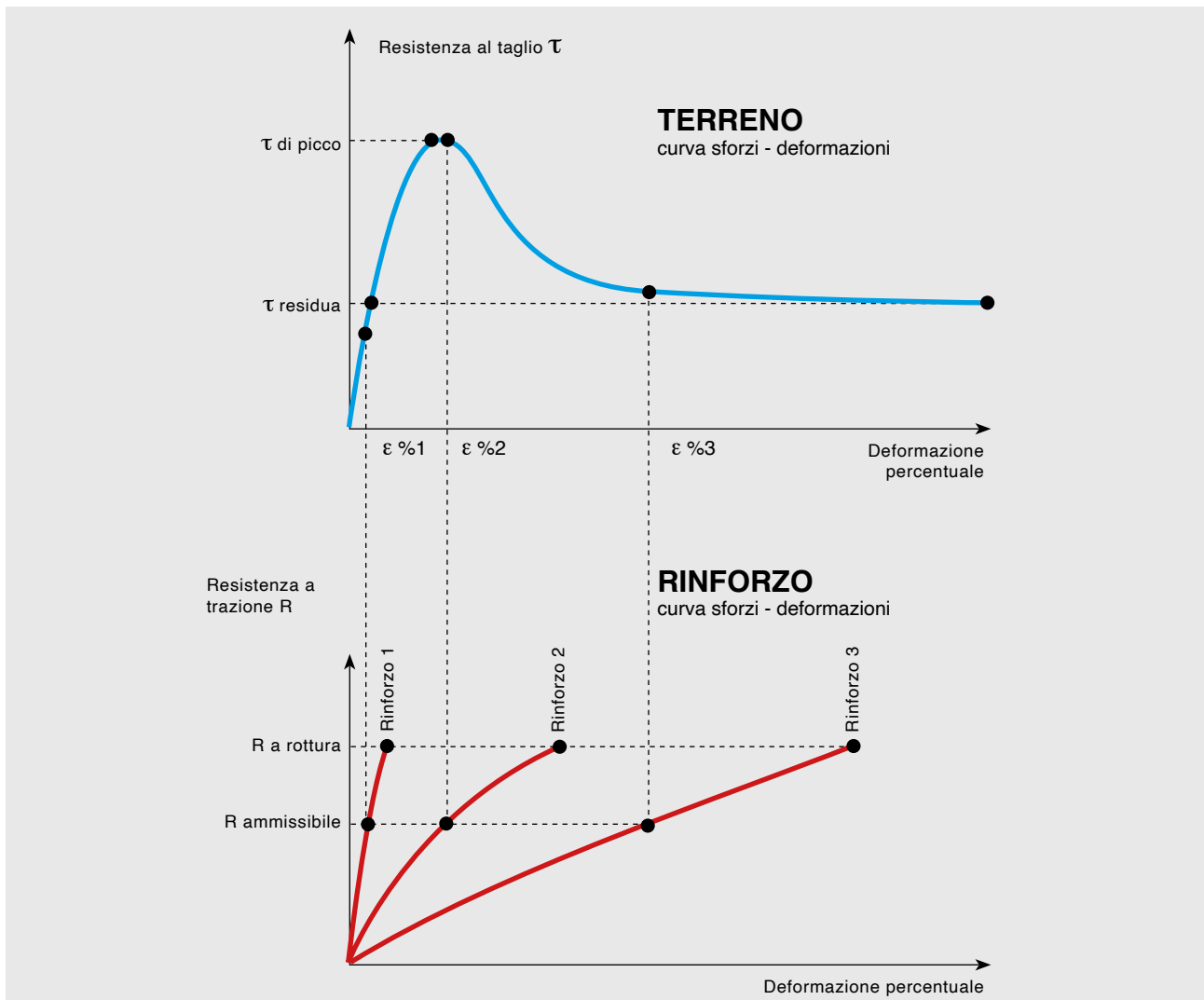
Fig. 4: Compatibilità deformativa terreno/rinforzo
