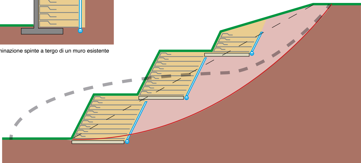
Ripristino di un pendio franato
