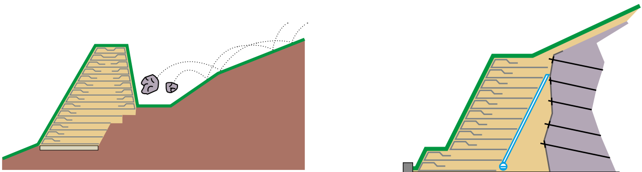
Vallo paramassi
