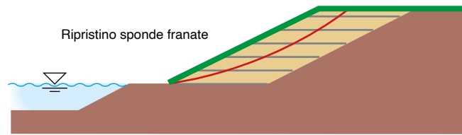
Argine fluviale
