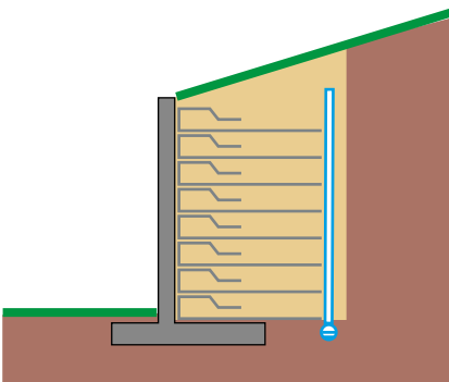
Eliminazione spinte a tergo di un muro esistente
