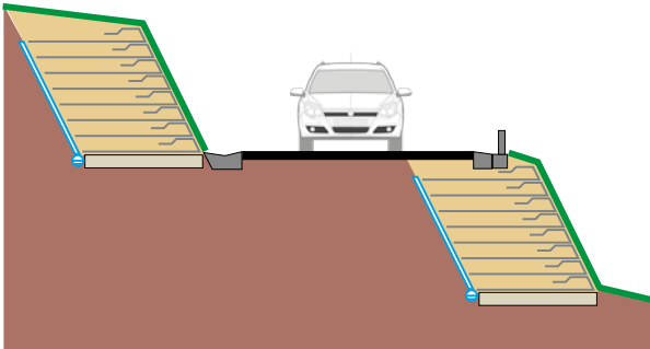
Opera di sostegno di controripa e sottoscarpa
