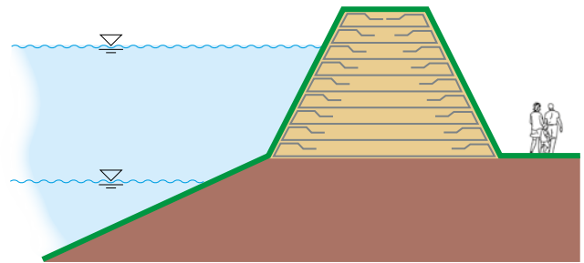
Argine fluviale
