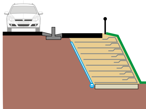
Ampliamento sede stradale
